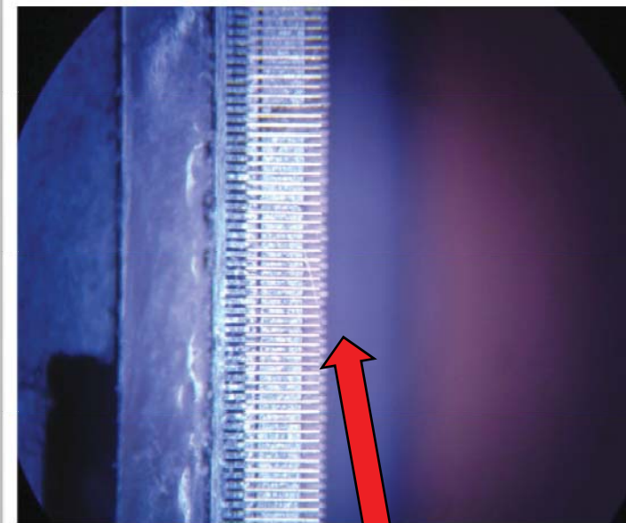
20μ±1μ超狭ピッチのエッチング加工を 実現化！！
